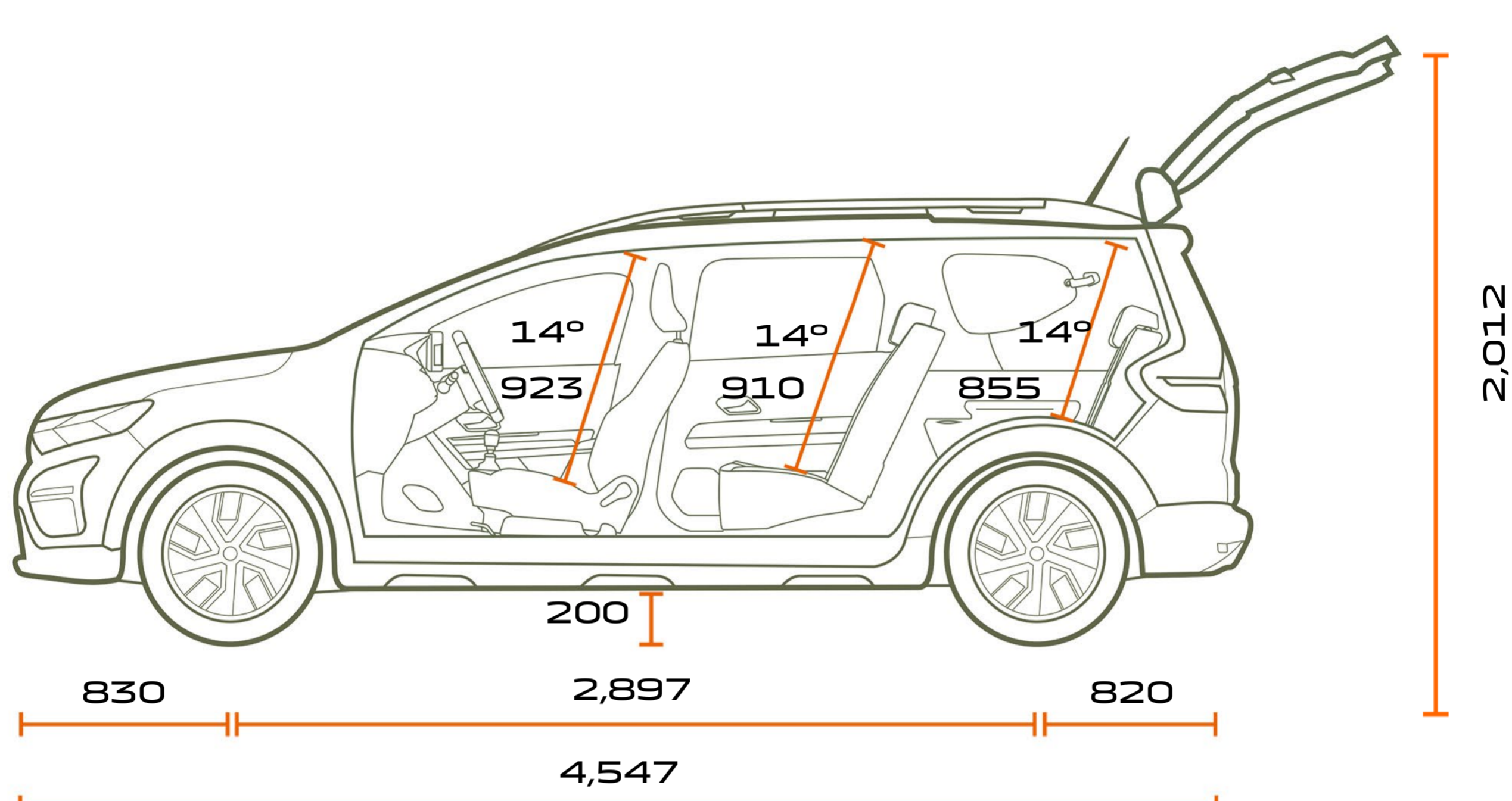
FRÅN SIDAN
